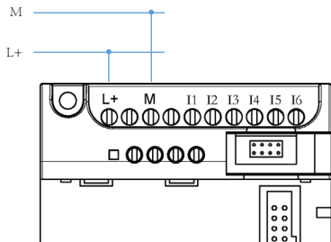
图 2.5 直流型
