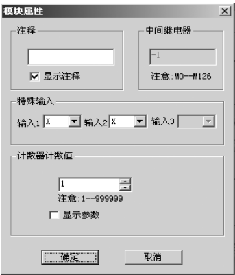
图 3.16 带有计数器的模块属性设置
