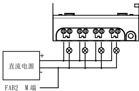
图 2.10 D 型晶体管输出
