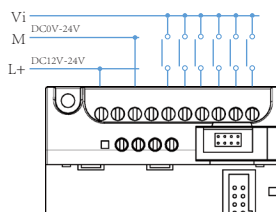
图 2.7 直流型
