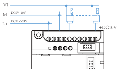
图 2.8 直流型 (D/GD 型)
