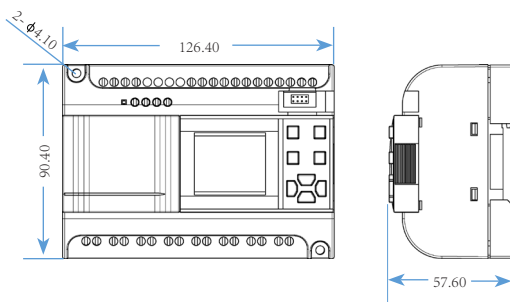
图 2.3 FAB2 20 点系列安装尺寸 (mm)
