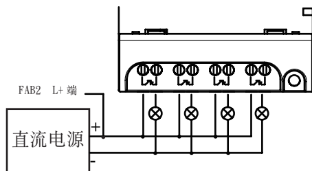
图 2.11 GD 型晶体管输出
