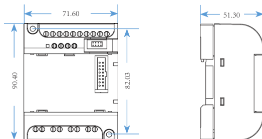
图 2.2 FAB2 10 点系列安装尺寸 (mm)
