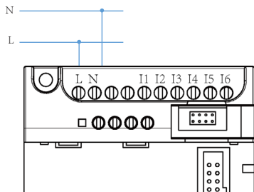
图 2.4 交流型
