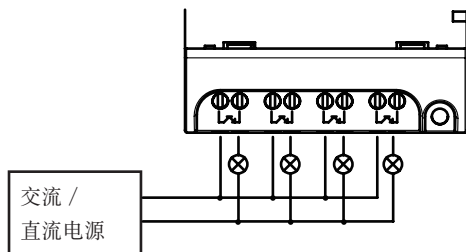
图 2.9 继电器输出
