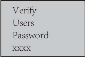
图 4.3 密码界面
