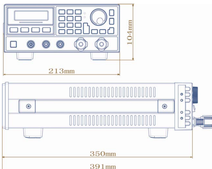
含套尺寸
