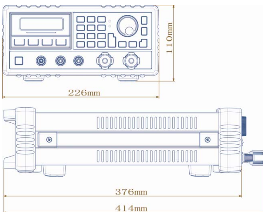
含套尺寸
